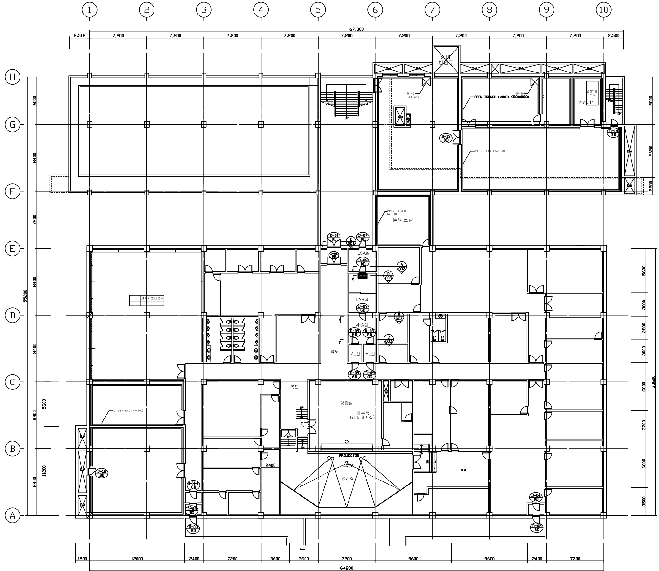
1 지하1층 화생방 설비 평면도 SCALE : 1/150
